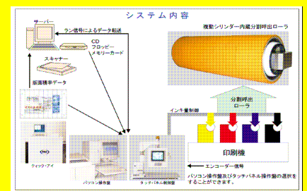
分割呼出コンピュータコントロールシステム(複動型)
